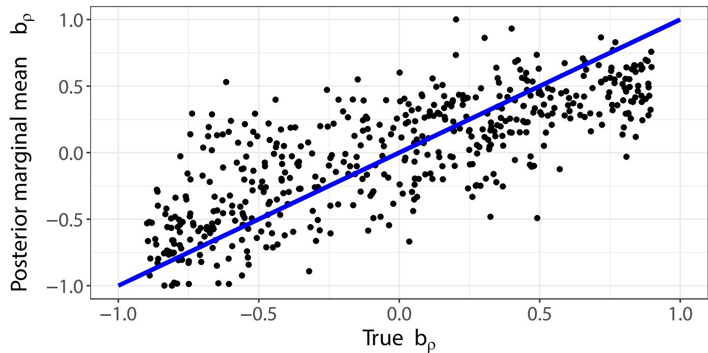
(d) Tipping process : b_\rho estimates vs true b_\rho
