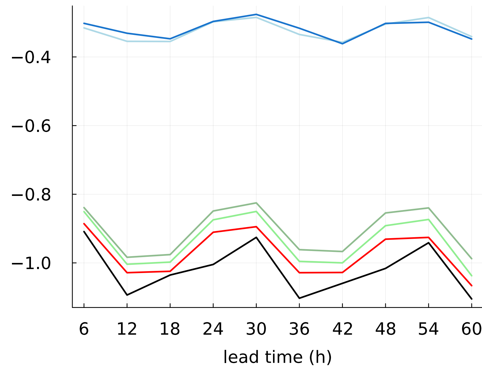
mean error ( \text{m s}^{-1} )
