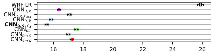
(d) u-component MAE ( \text{m s}^{-1} )
