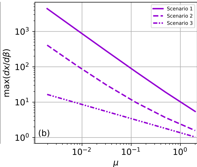
Cubic ODE
