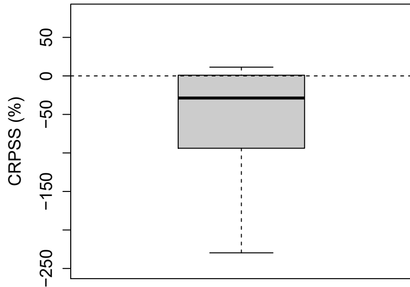
(d) 1 RAINR>0, 1 SNOWR>0, obs>1cm [14.7%]
