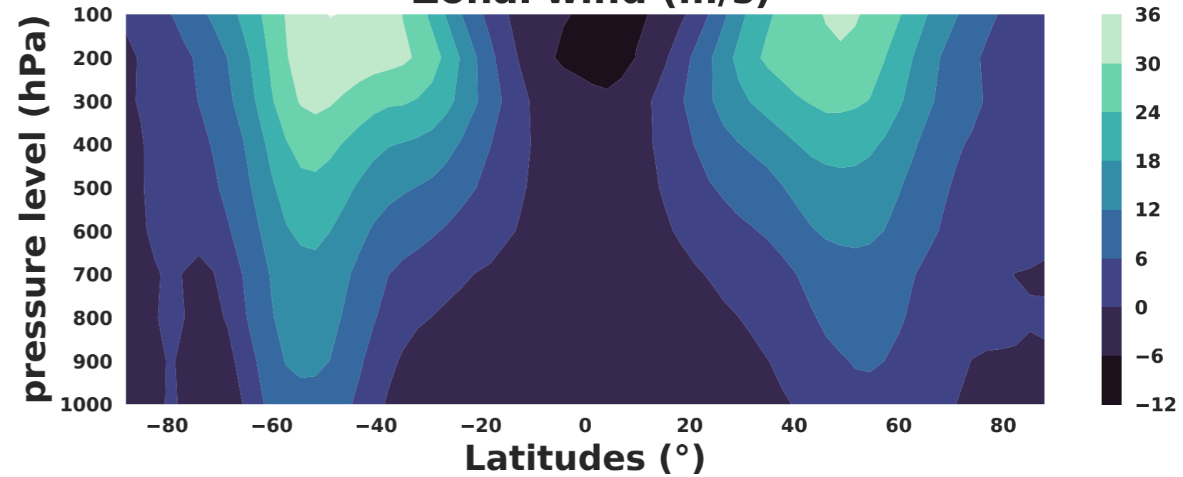
(d) Zonal wind (m/s)
