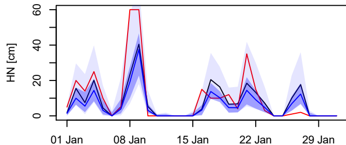
(d) + 72 h, station: 73023401, CRPSS: 20.96 %
