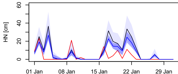
(b) + 24 h, station: 73235400, CRPSS: -19.17 %
