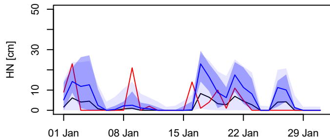
(d) + 96 h, station: 73235400, CRPSS: 35.01 %
