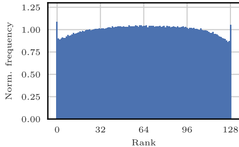
(d) S(\text{IT}_s \text{P}_{\text{RK}})^{\times R}
