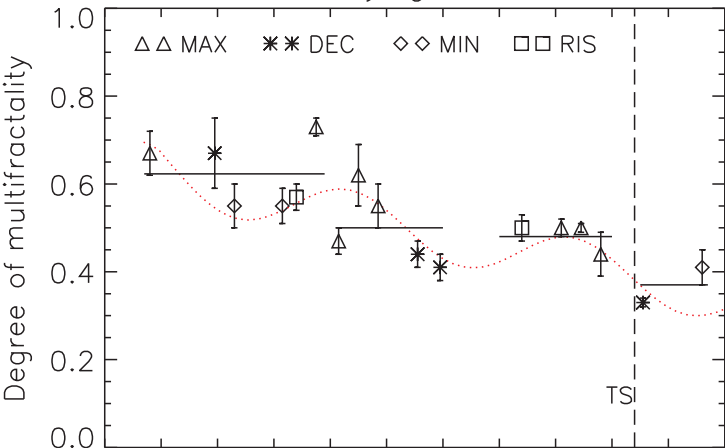
Voyager 1
