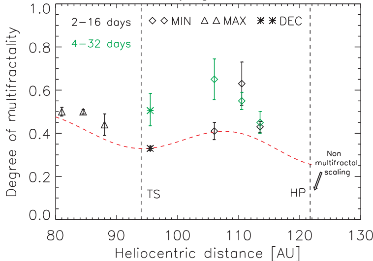
Voyager 1
