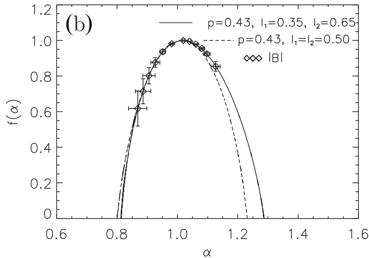
V2 2008, 1–256, R = 85–88 AU
