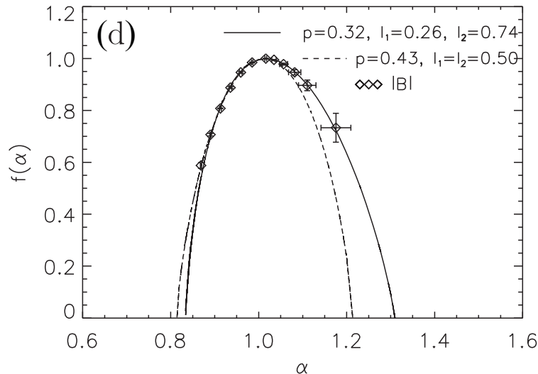
V2 2009, 1–256, R = 88–90 AU
