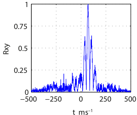
(i) FLOC, GSNR = 15 dB
