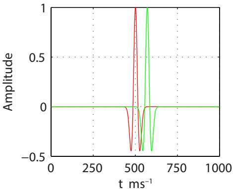
(d) GCC, GSNR = 0 dB
