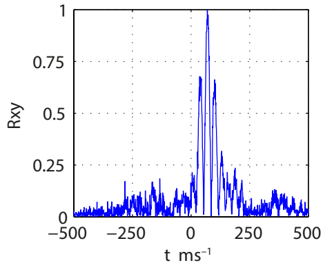
(i) FLOC, GSNR = 15 dB
